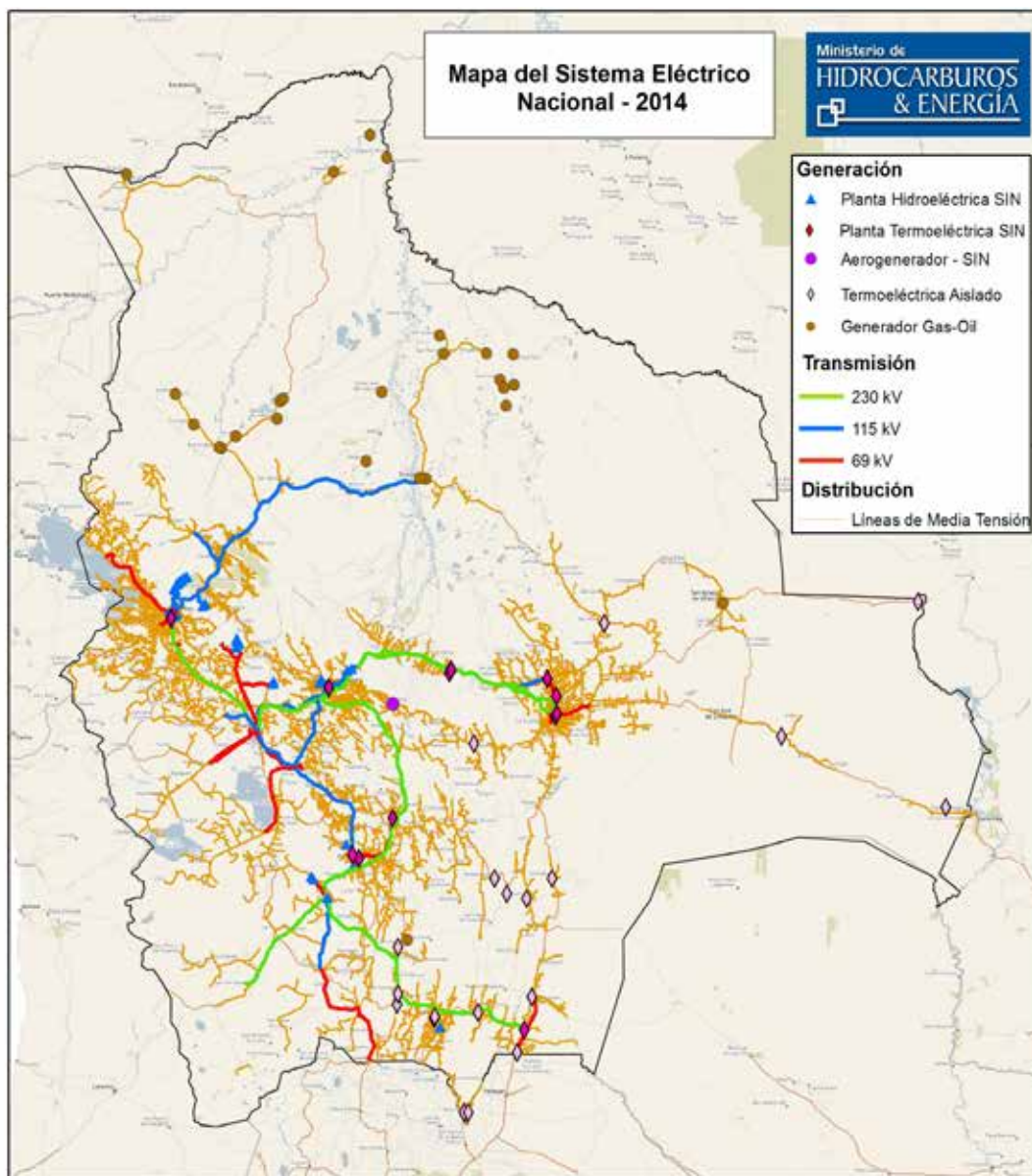
Figura 6. Mapa General del Sistema Eléctrico Nacional
