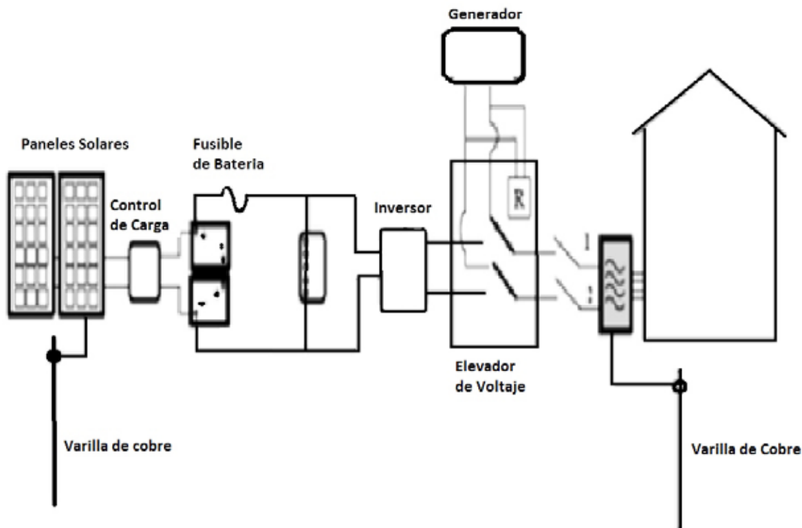
Diagrama de un sistema fotovoltaico híbrido
