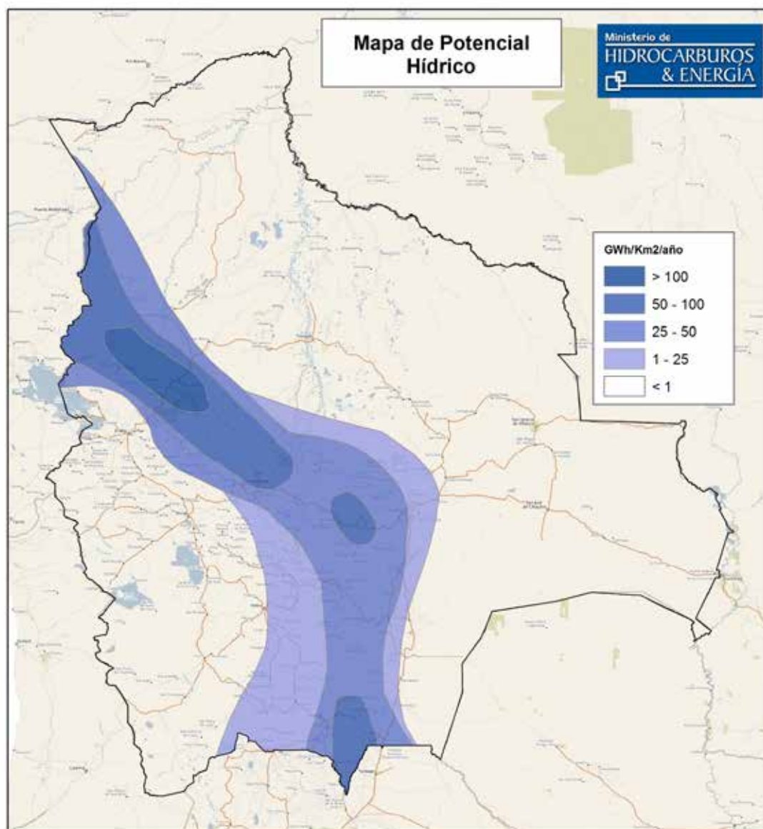
Figura 13. Potencial hídrico
